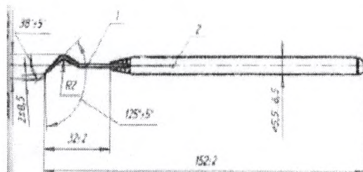
Рисунок 7 – Зона стоматологический тип F (061) с пластмассовой ручкой.
