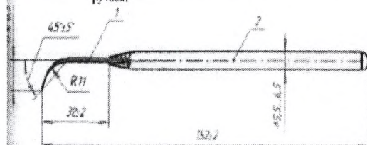
Рисунок 8 – Зона стоматологический тип G (071) с пластмассовой ручкой.
