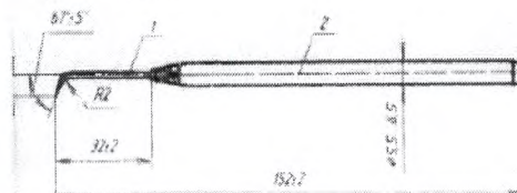
Рисунок 5 – Зона стоматологический тип D (041) с пластмассовой ручкой.
